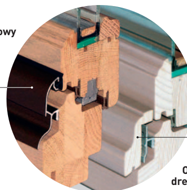
Softline Prestige XL Szerokość systemu 78 mm.
